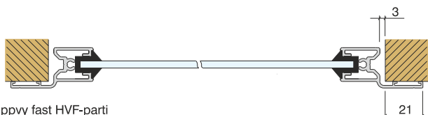
Toppvy fast HVF-parti
