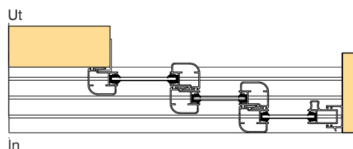
Förlängd spårskena höger 3-del
