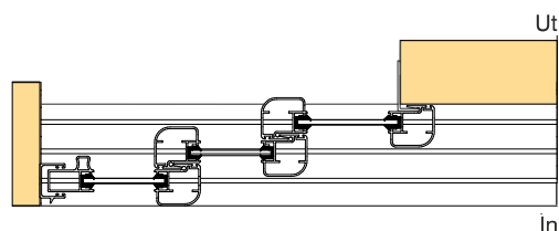
Förlängd spårskena vänster 3-del
